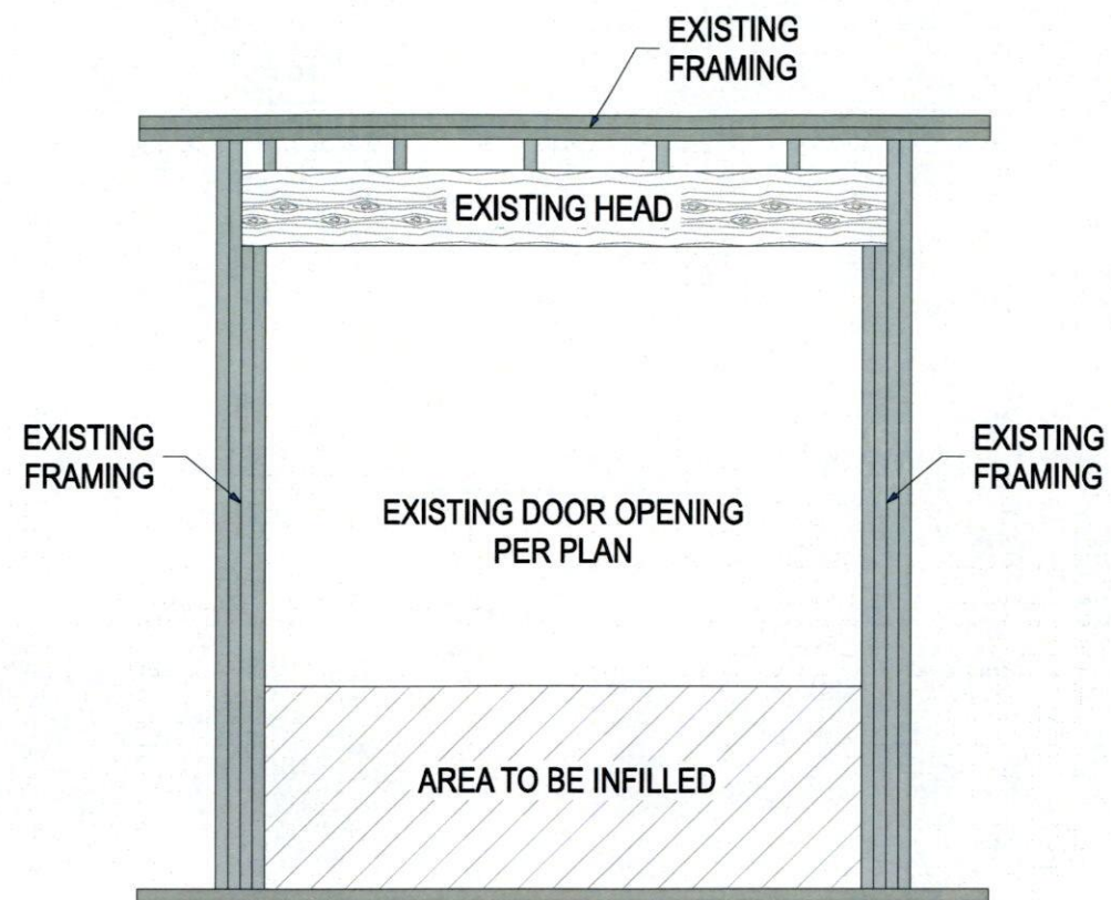
EXISTING DOOR FRAMING SCALE: N.T.S.
