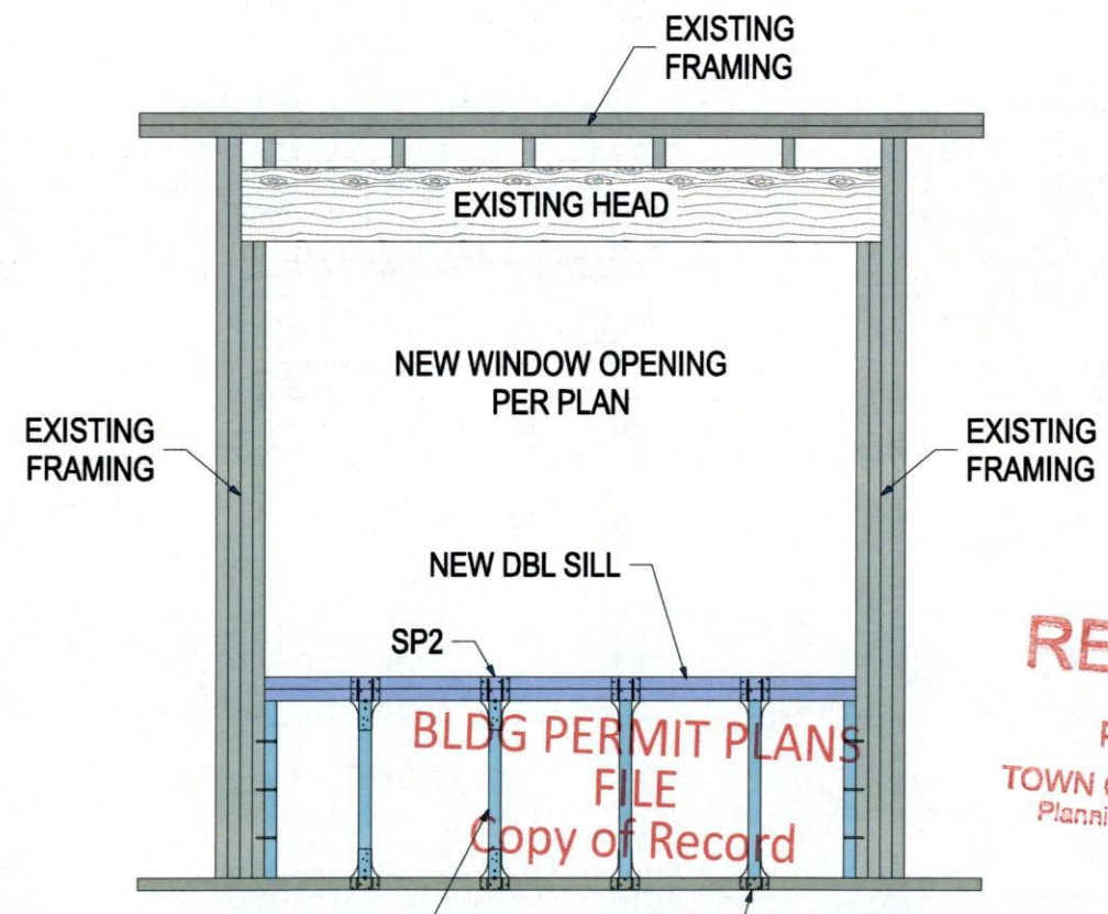
NEW WINDOW FRAMING SCALE: N.T.S.
