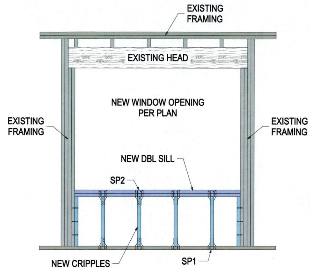
NEW WINDOW FRAMING SCALE: N.T.S.
