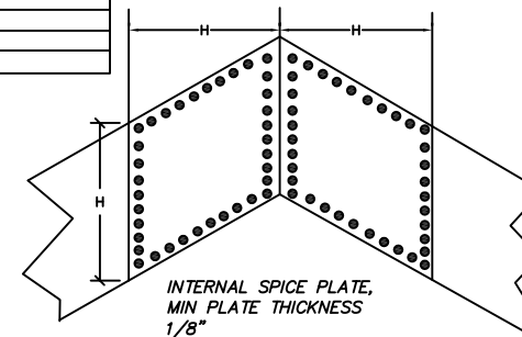
INTERNAL GUSSET DETAIL SCALE N.T.S.
