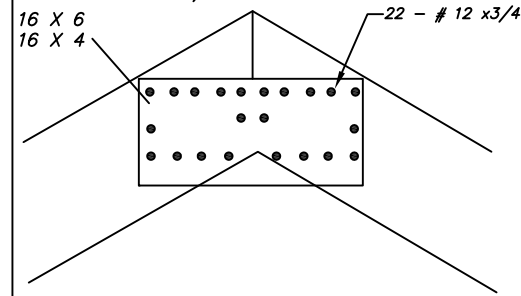
EXTERNAL GUSSET DETAIL SCALE N.T.S.
