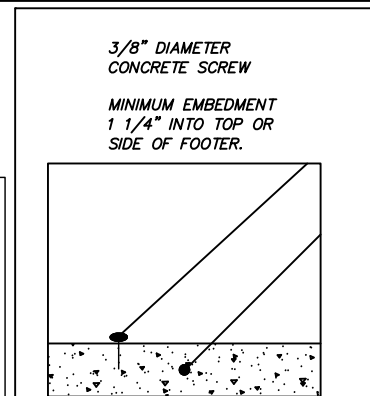
CABLE TO FOOTER SCALE N.T.S.
