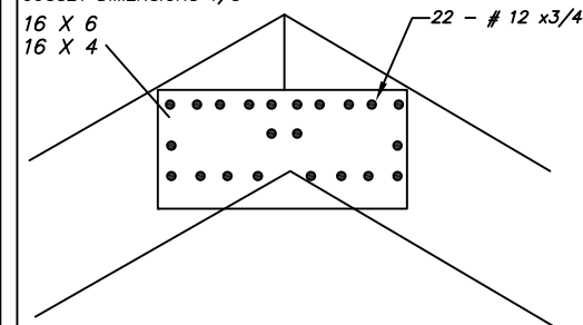
EXTERNAL GUSSET DETAIL SCALE N.T.S.
