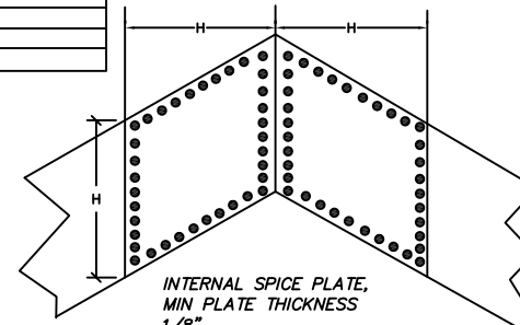
INTERNAL GUSSET DETAIL SCALE N.T.S.
