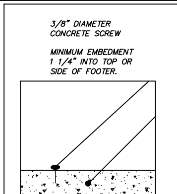
CABLE TO FOOTER SCALE N.T.S.
